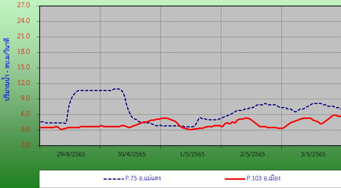
กราฟแสดงปริมาณน้ำปิ้งรายชั่วโมงรอบวันที่ 17/2565 ที่สถานีแม่ น้ำปิ้ง (P.75) บ้านซ้อแล อ.แม่แตง และที่สถานีแม่ น้ำปิ้ง(P.103) บ้านป่าซ่อยใต้ อ.เมือง จ.เชียงใหม่
